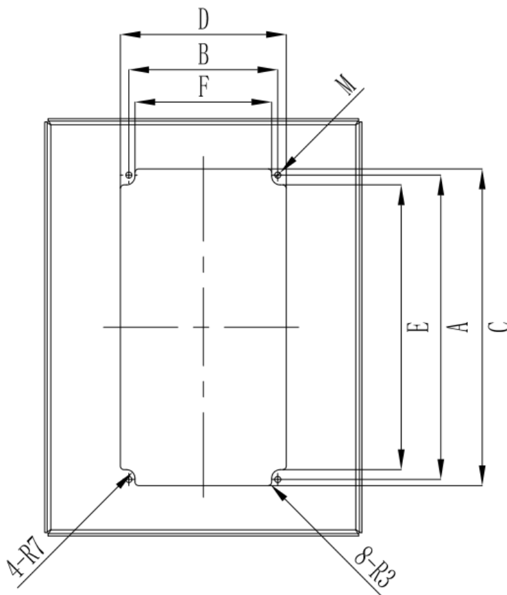
图 3-5 塑胶结构 11-14 机型嵌入式安装板示意图
