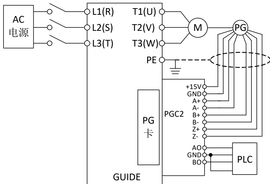
PGC2 卡接线原理示意图:
