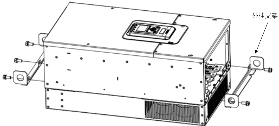
图 3-2 钣金结构安装外挂支架示意图
