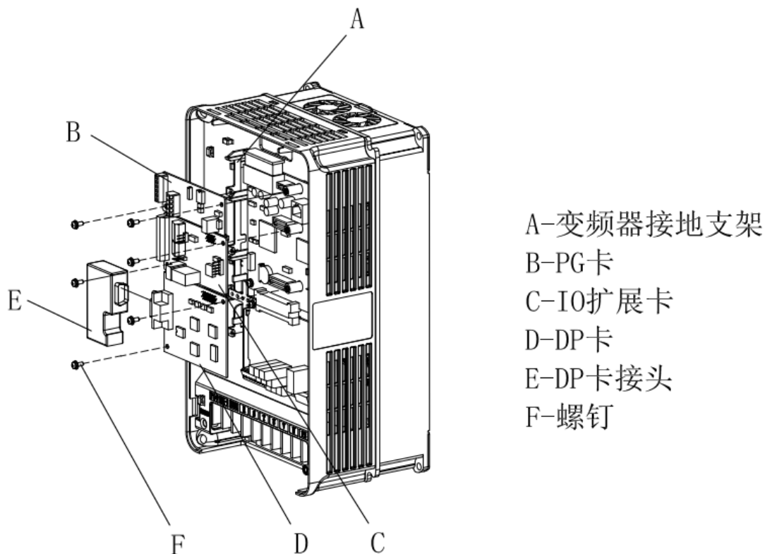
37kW 及以下变频器附件卡的安装
