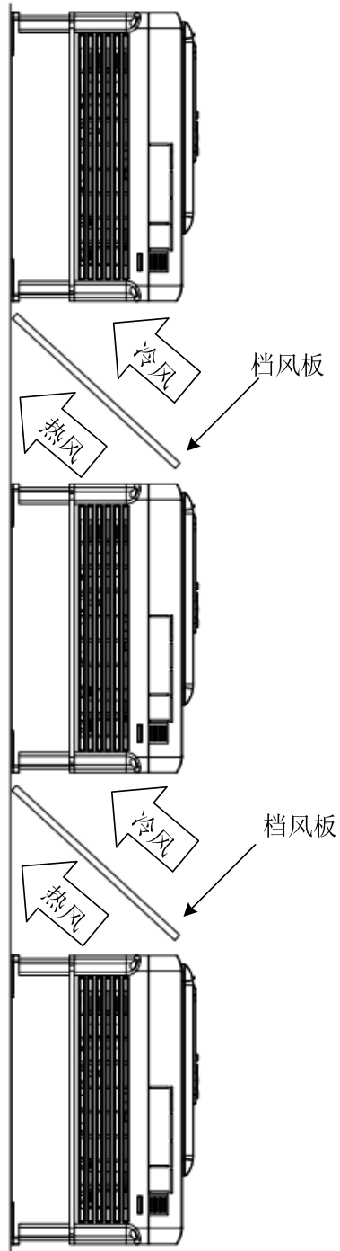
图 3-8 垂直安装示意图
