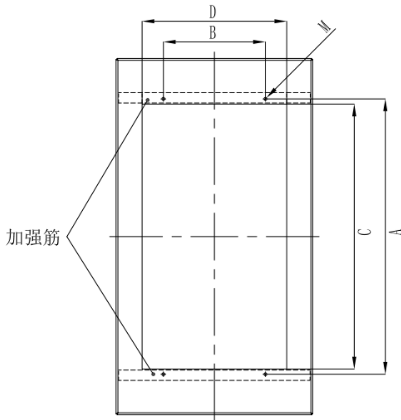
图 3-6 钣金结构 15-16 机型嵌入式安装板示意图
