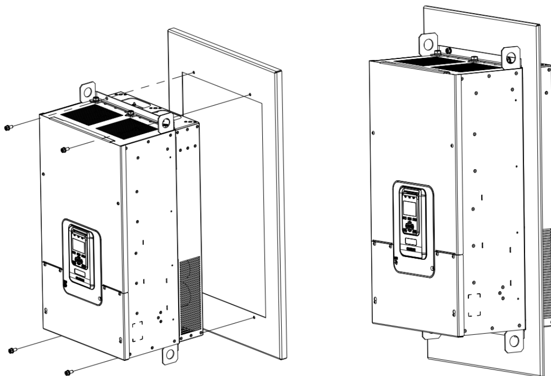
图 3-3 钣金结构嵌入式安装示意图和效果图
