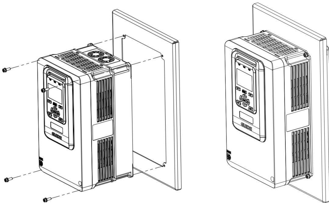
图 3-4 塑胶结构嵌入式安装示意图和效果图
