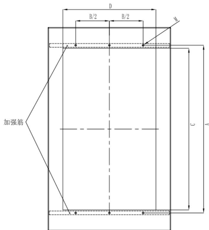
图 3-7 钣金结构 17-19 机型嵌入式安装板示意图
