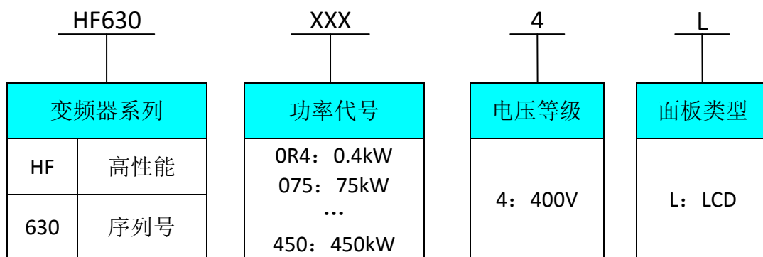
图 2-1 产品型号含义
