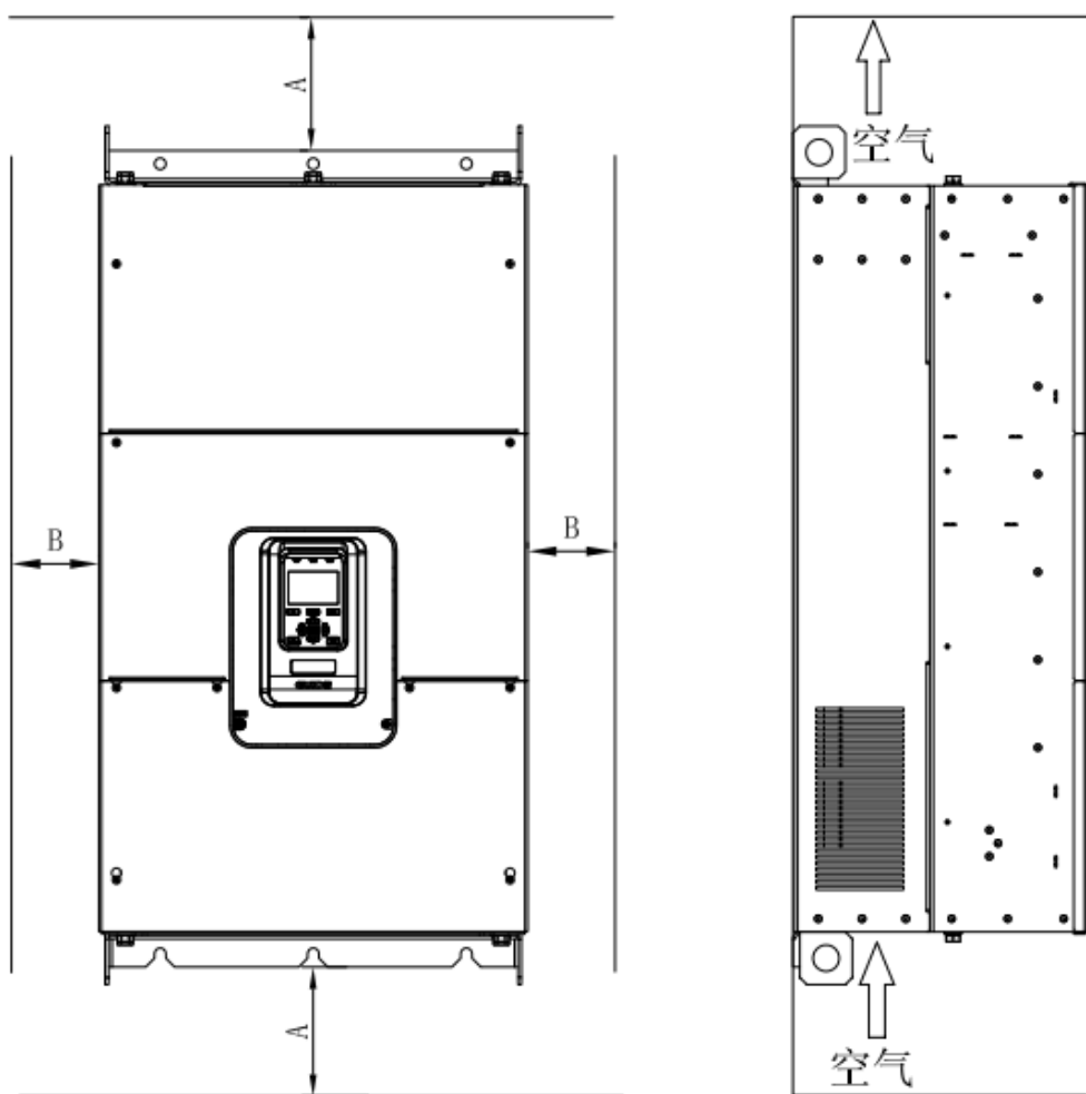
图 3-1 壁挂式安装
