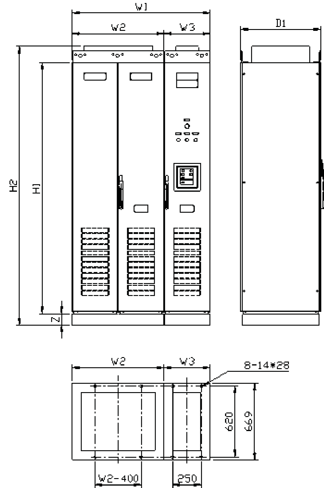
整流回馈HF500A-160-6-C+P、HF500A-250-6-C+P、HF500A-315-6-C+P和HF500A-500-6-C+P成柜外形示意图
