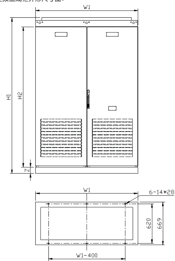
D5~D6机型示意图
