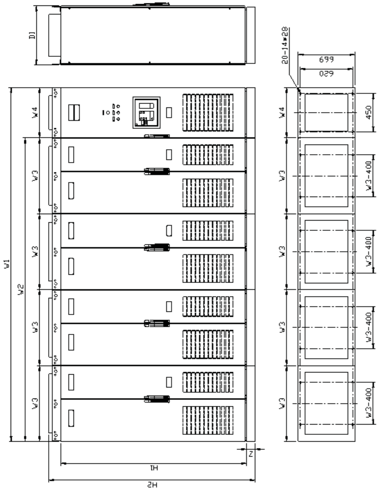
整流回馈HF500A-2000-6-C+P成柜外形示意图
