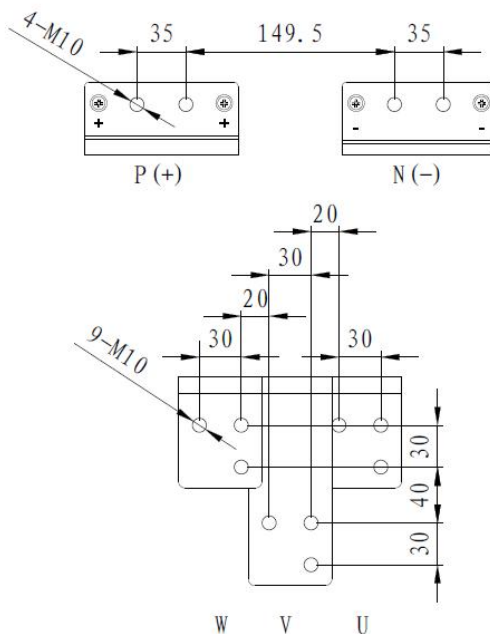
HF650B-400-4-D 主接线端子示意图
