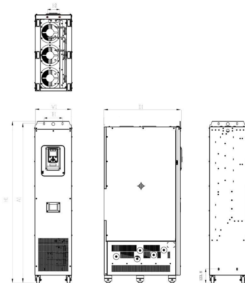
逆变器(160kW~400kW)外形示意图
