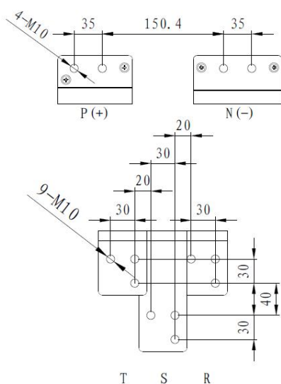
HF650A-250-4-D 主接线端子示意图
