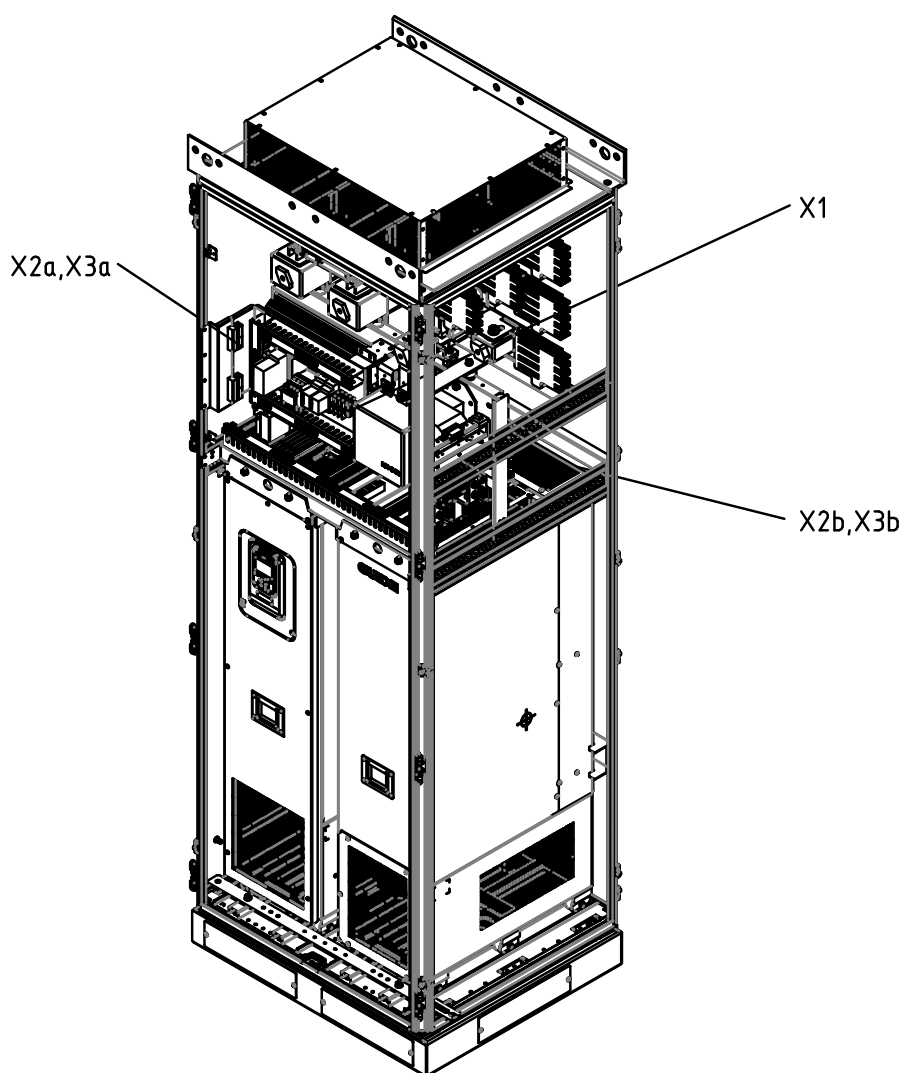
整流回馈2标准成柜（从柜）接线端子位置示意图（b）
