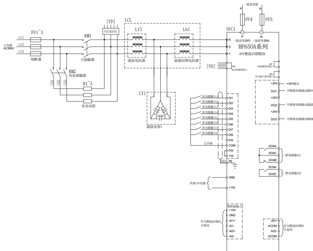
整流回馈单元的单机接线图
