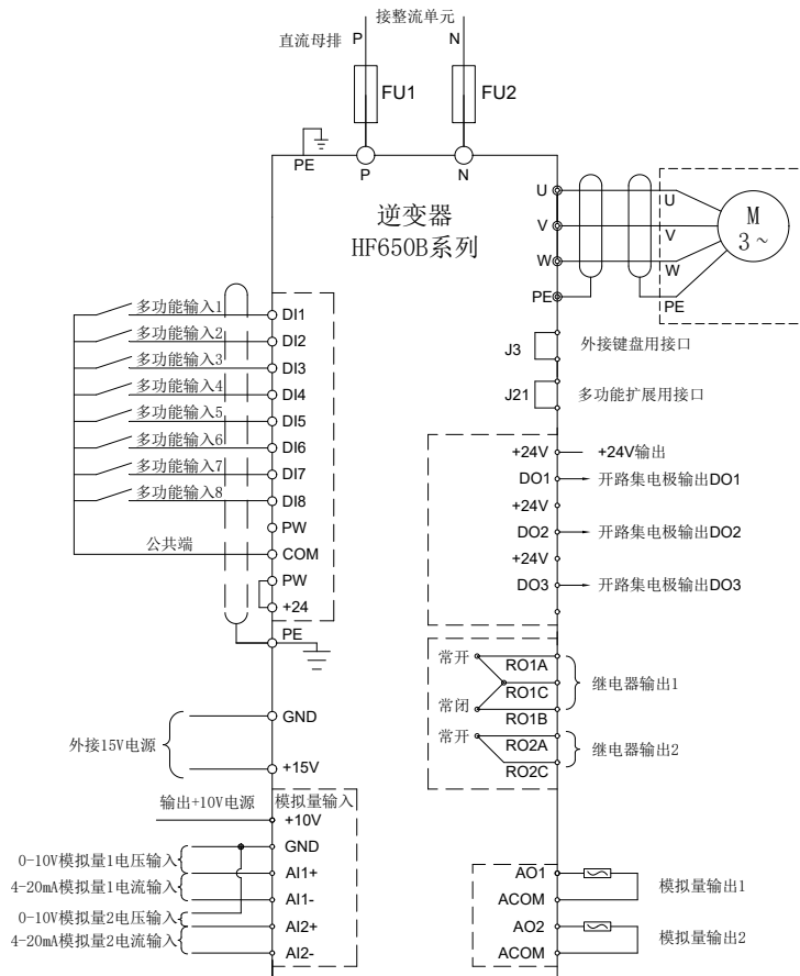
逆变器产品的单机接线图
