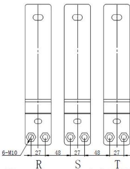
HF650A-250-4-D LCL 主接线端子示意图
