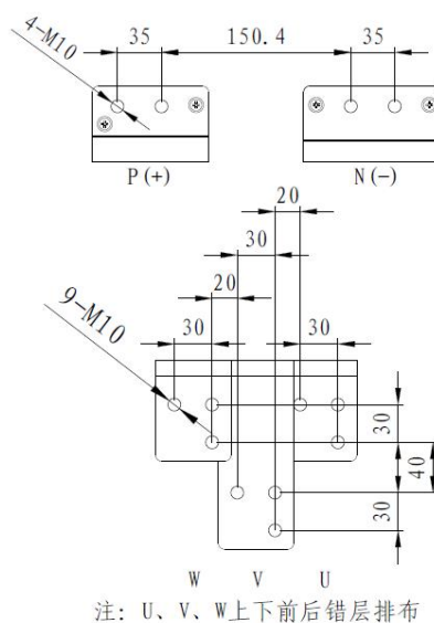
HF650B-250-4-D 主接线端子示意图
