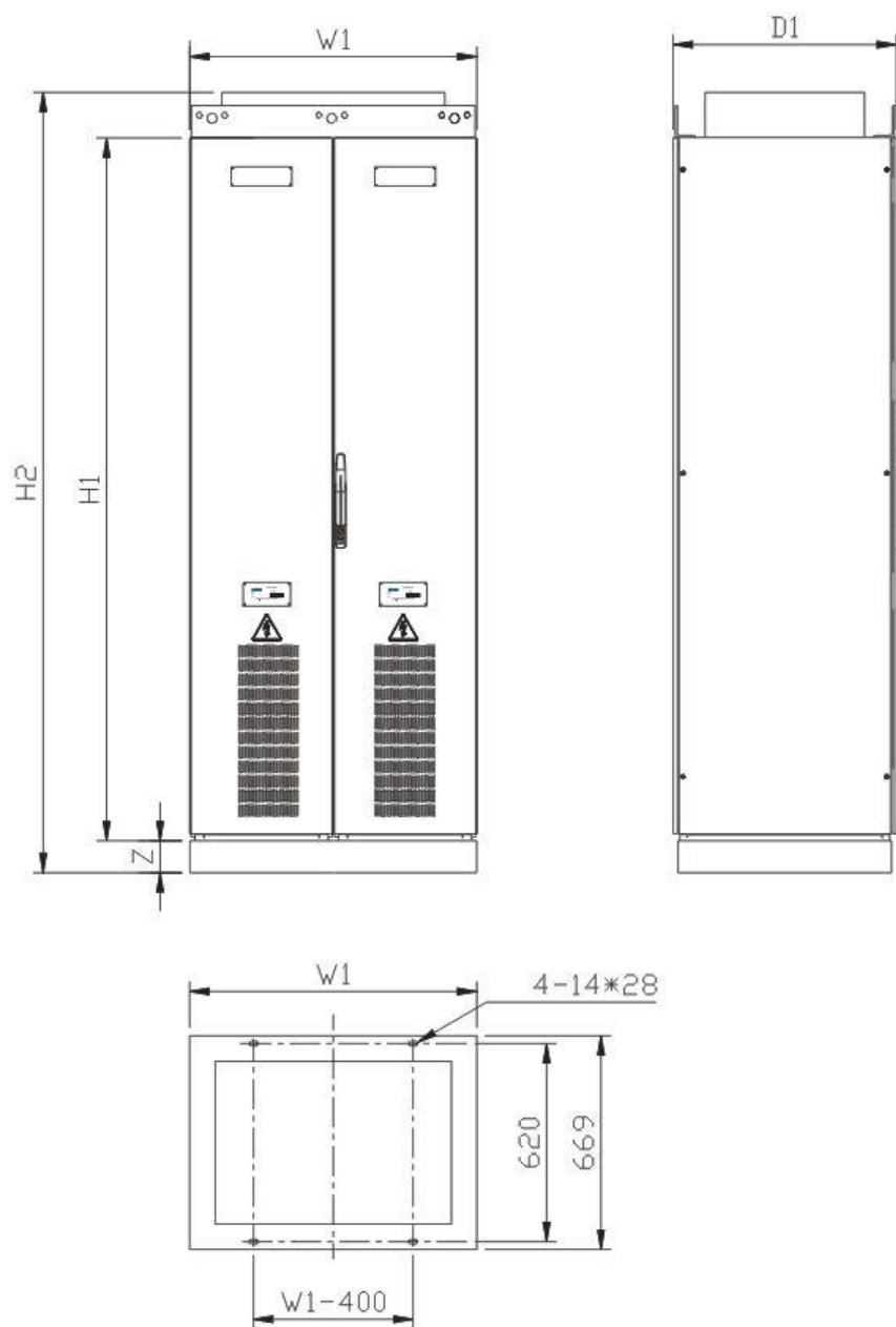
逆变器外形示意图
