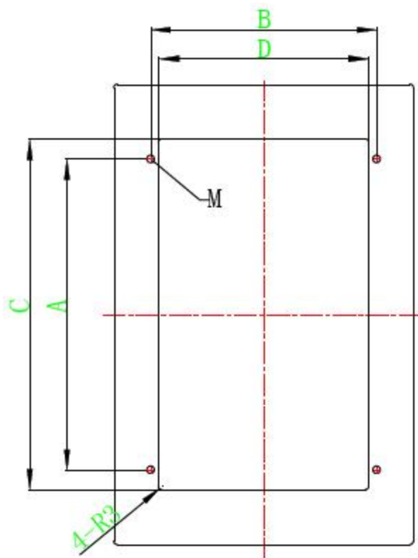
图 3-6 塑胶结构 13 机型嵌入式安装板示意图
