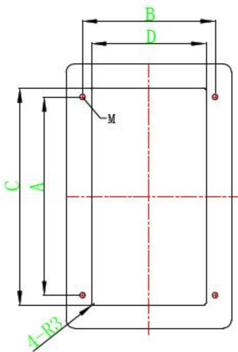
图 3-5 塑胶结构 11-12 机型嵌入式安装板示意图
