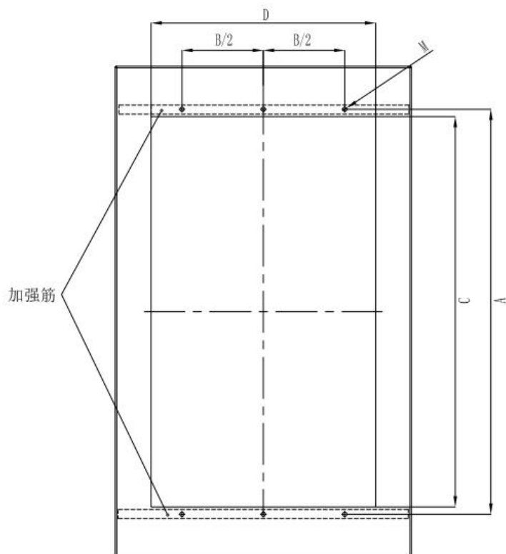
图 3-9 钣金结构 17-19 机型嵌入式安装板示意图
