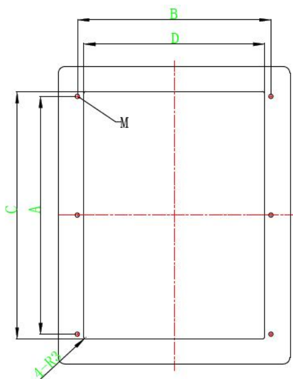
图 3-7 塑胶结构 14 机型嵌入式安装板示意图
