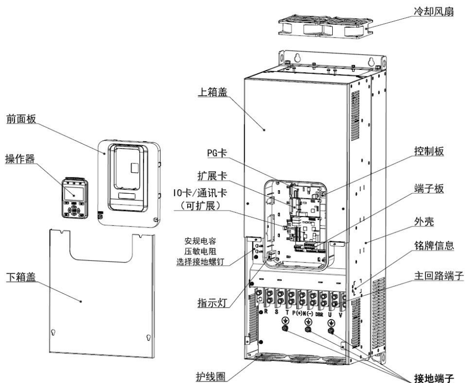
N6 产品部件示意图 (三相 380V~480V, 90kW)
