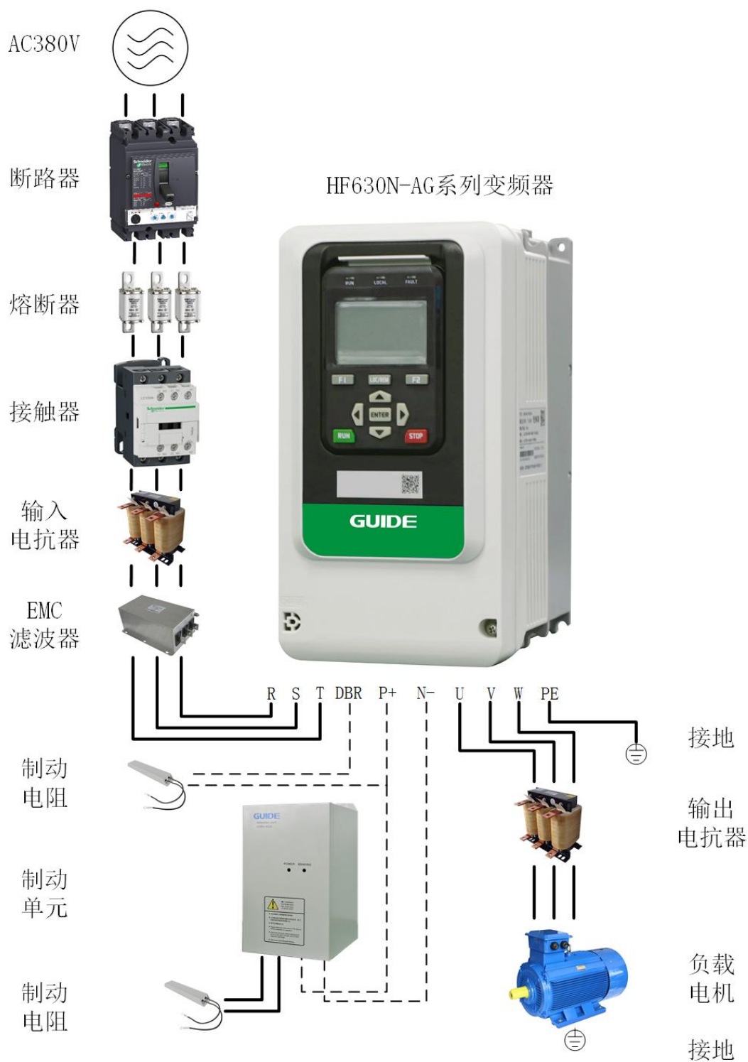
HF630-AG 变频系统外围电气元件的使用说明
