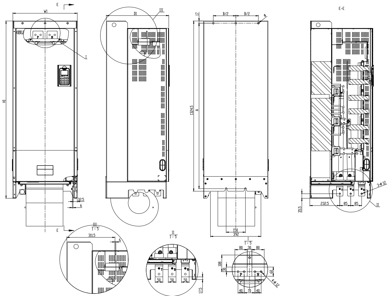
整流回馈 HF500A-315-4-D 和 HF500A-400-4-D 外形示意图
