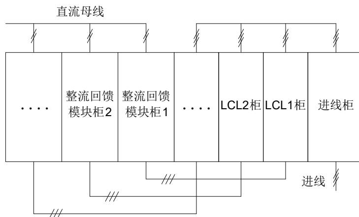
整流回馈单元的配线规格说明：
