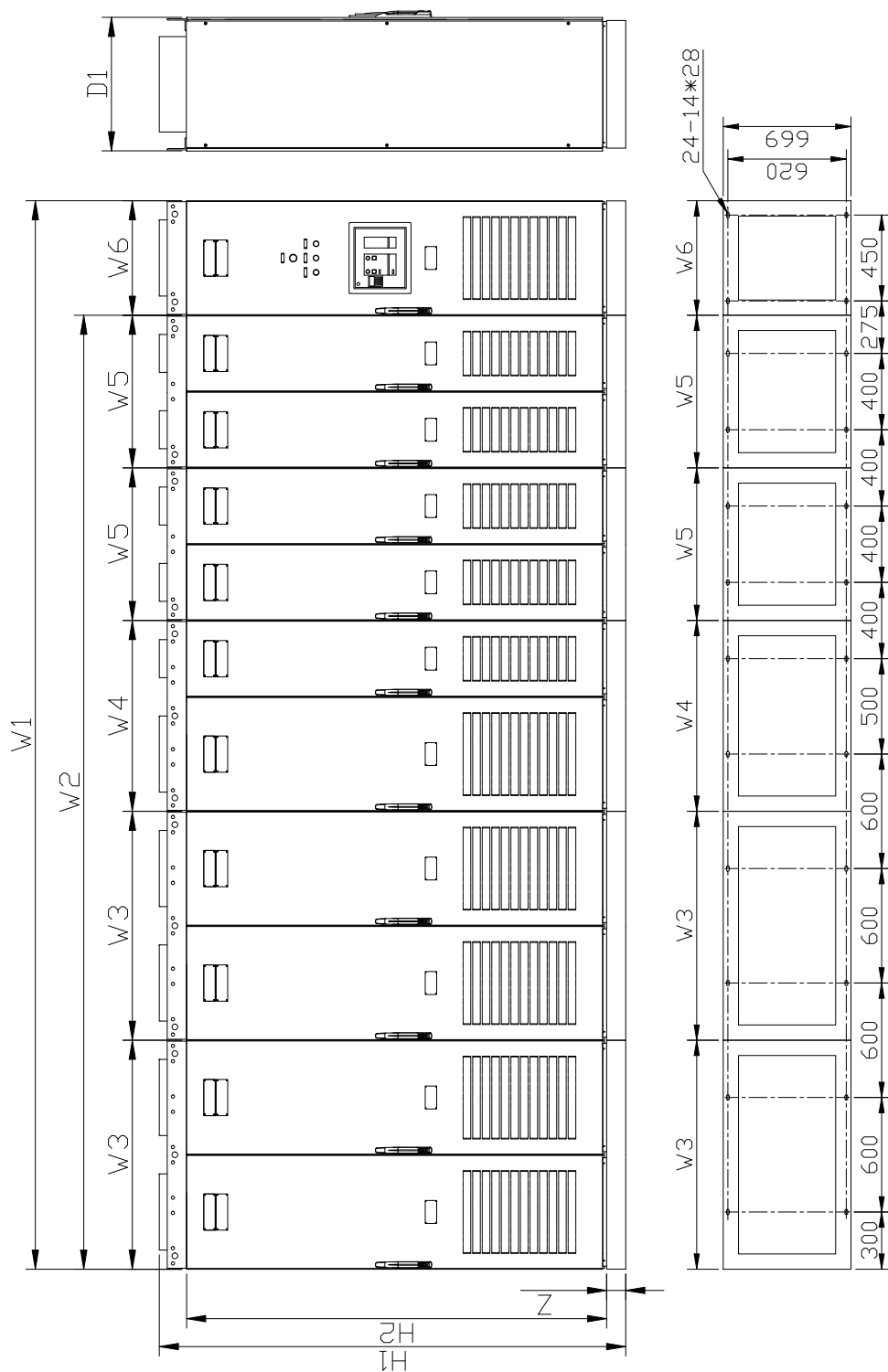
整流回馈 HF500A-2000-4-C 成柜外形示意图
