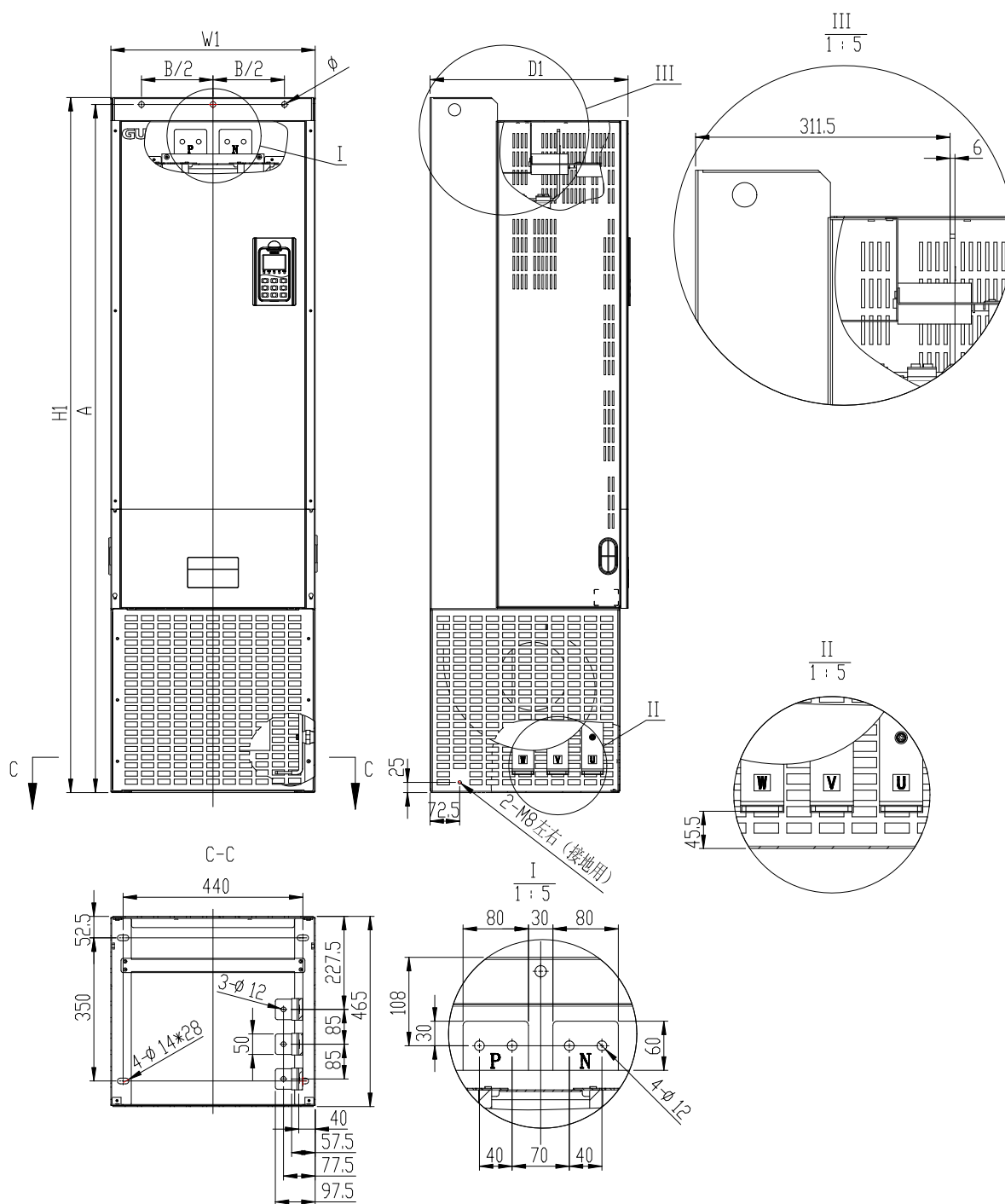
逆变器 HF500B-315-4-D、HF500B-355-4-D 和 HF500B-400-4-D 外形示意图
