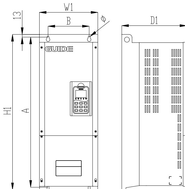
逆变器 HF500B-037-4-D、HF500B-045-4-D 和 HF500B-055-4-D 外形示意图
