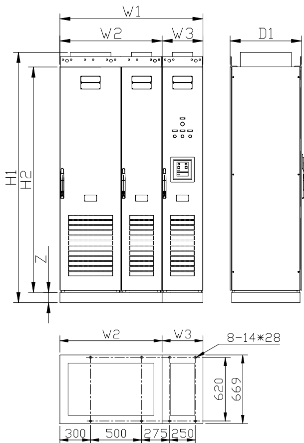
整流回馈 HF500A-250-4-C、HF500A-315-4-C 和 HF500A-400-4-C 成柜外形示意图
