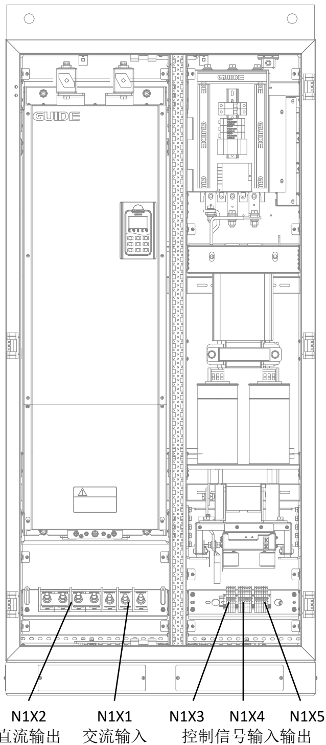
整流回馈 400kW 及以下 C1~C4 成柜产品接线端子位置示意图
